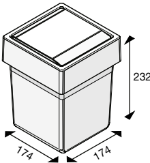
Contenedor de tapa bandeja
