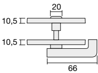
Desbloqueo exterior con señalizador libre-ocupado con roseta de Ø65 mm. y tornillos ocultos. Fijación mediante tornillos pasanteas.
