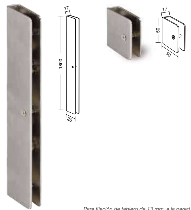
Para fijación de tablero de 13 mm. a la pared.
