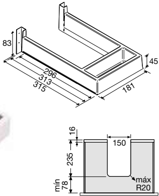
Salvasifón con compartimento
