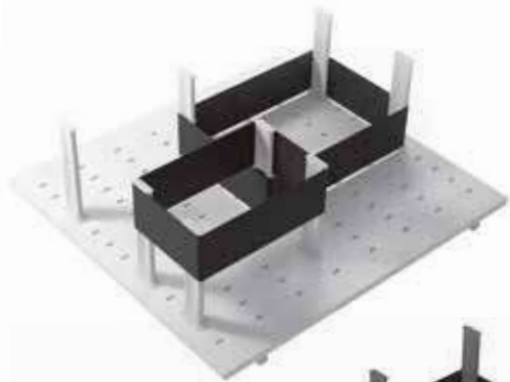
Instalación con escurridor y montaje sin gomas organizadoras
