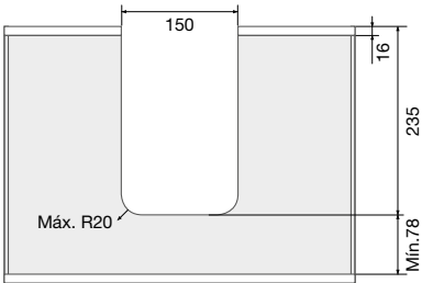
Mecanizado del cajón.
