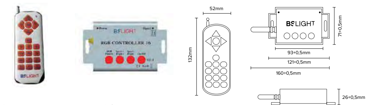
Controlador para bombillas16 / Controller for bulb16
