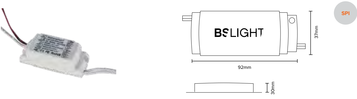
AMPLIFICADOR PARA TIRA DIGITAL SPI
